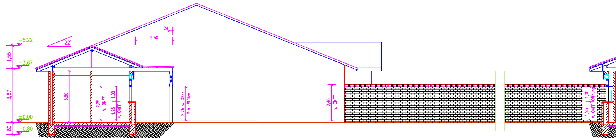
Schnitt "Abschuss" / Ziel Schießstand
